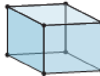
Monoclinic
