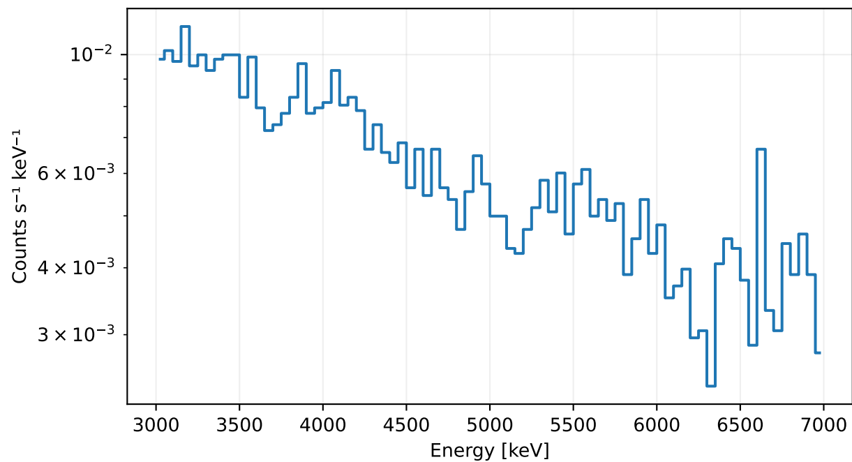
3000–7000 keV, 50 keV bins
