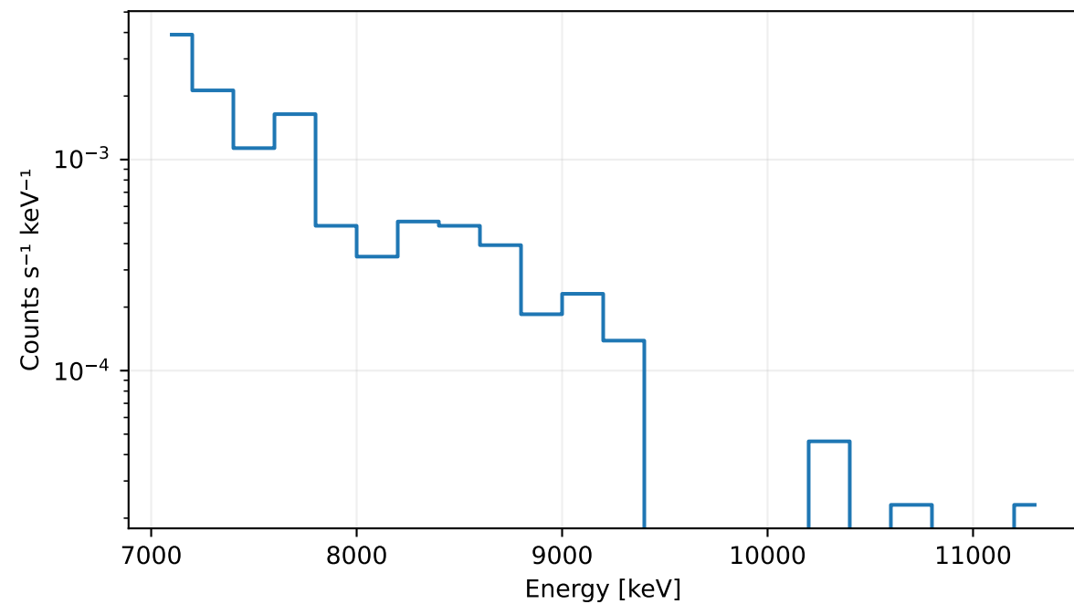
7000–11400 keV, 200 keV bins
