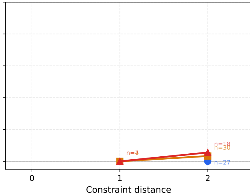
gpt-4.1-mini
