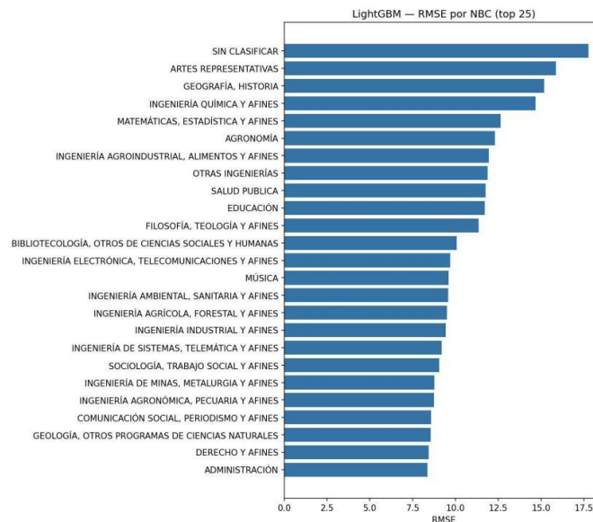
Figura 5. LightGBM — RMSE por Núcleo Básico del Conocimiento (top 25). Sin Clasificar y Artes Representativas concentran los errores más altos por alta heterogeneidad interna.
