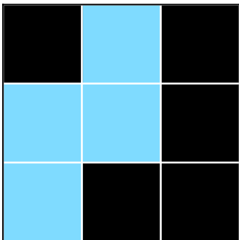
d631b094 — input
