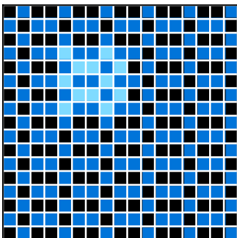
32597951 — input
