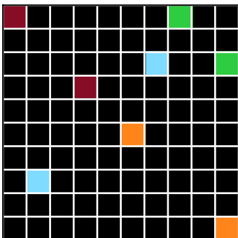
1f876c06 — input
