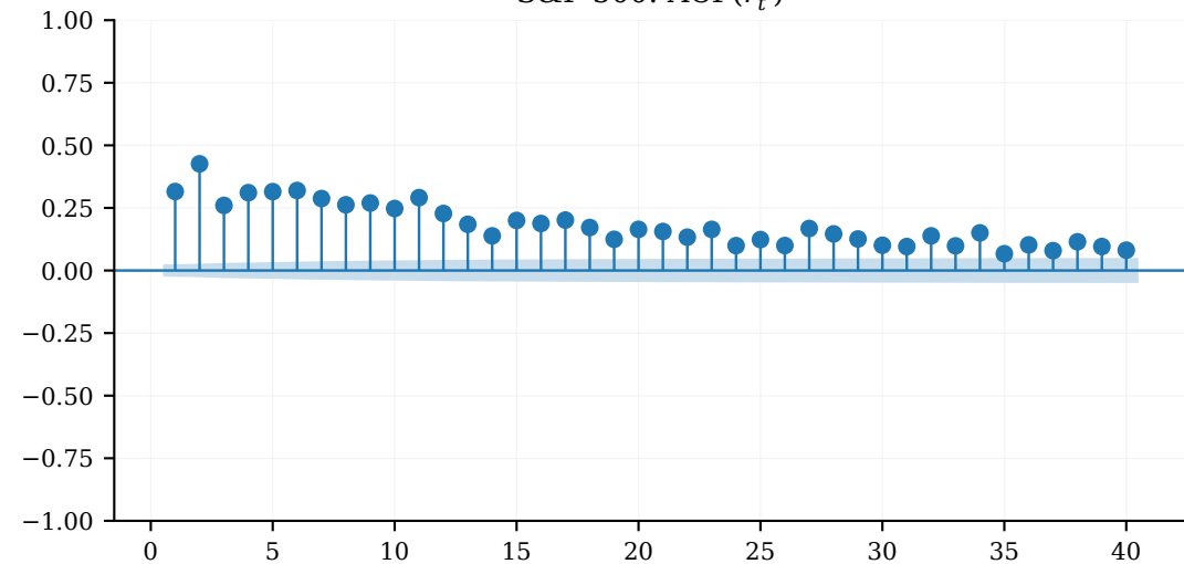
Oil: ACF(r_t^2)
