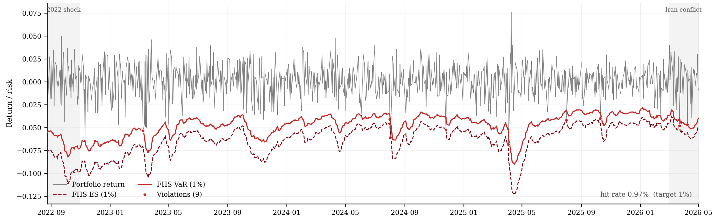
GRU (Student-t): one-step-ahead FHS VaR/ES
