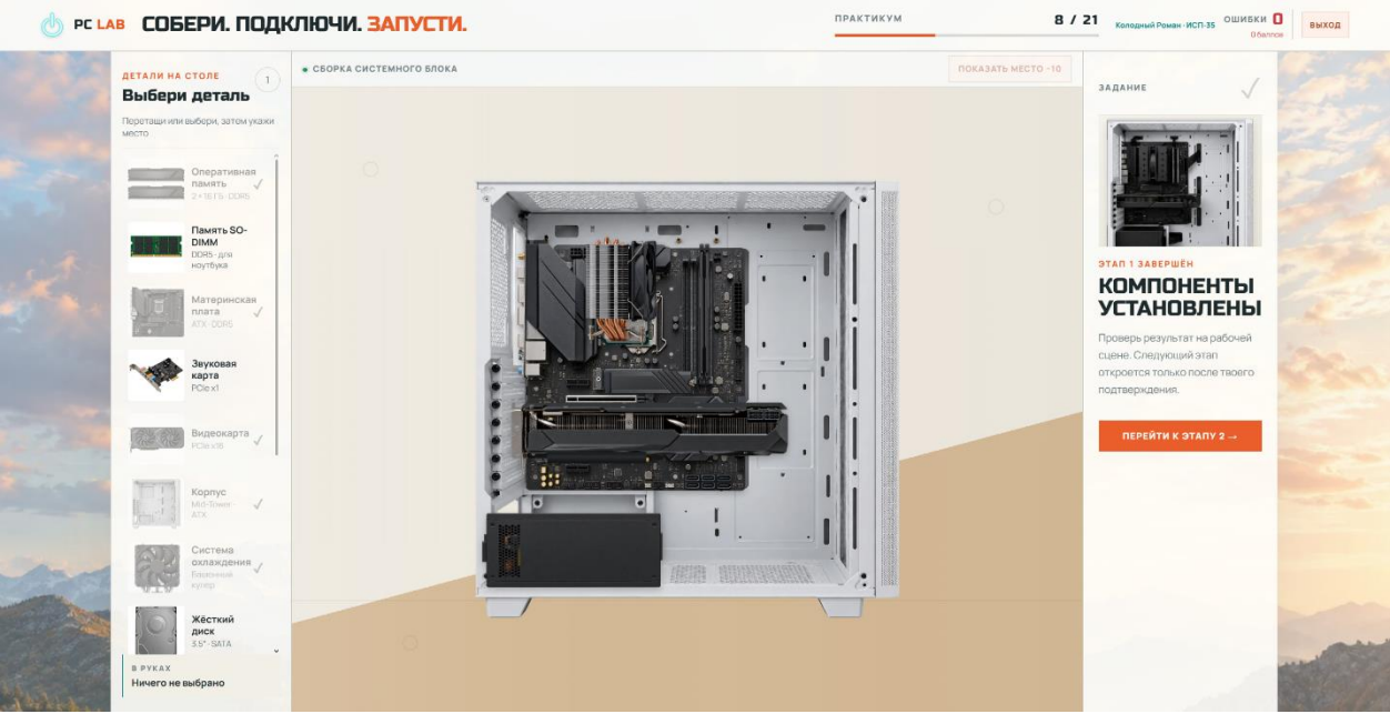
Скриншот 1
