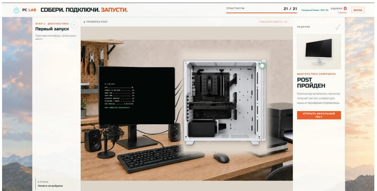
Скриншот 4
