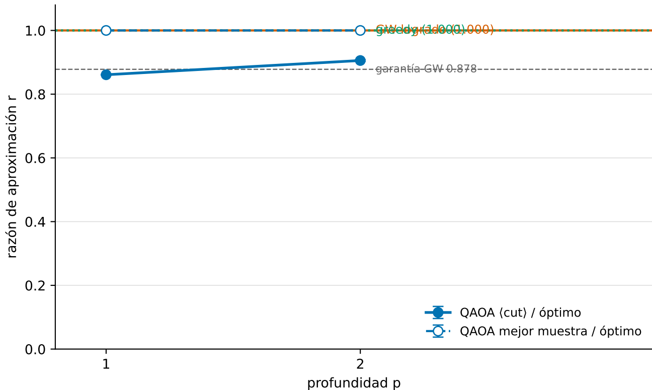
cr8-uniforme: QAOA vs líneas base clásicas (media \pm \sigma , 2 semillas)
