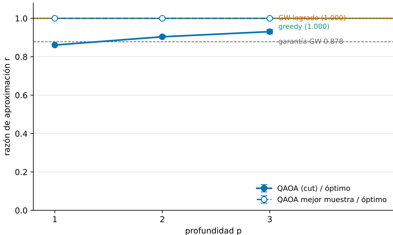
cr8-uniforme: QAOA vs líneas base clásicas (media \pm \sigma , 5 semillas)
