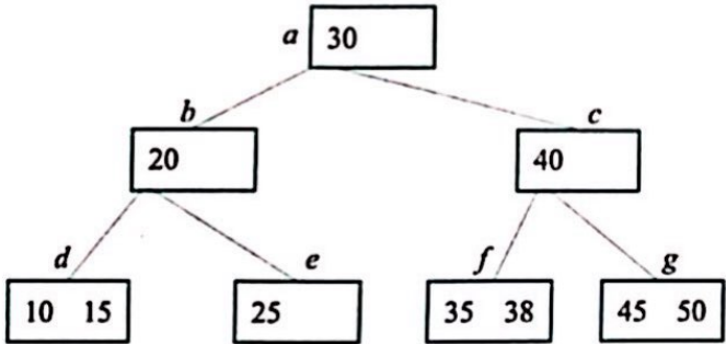
图 14-20 3 阶 B 树图示
