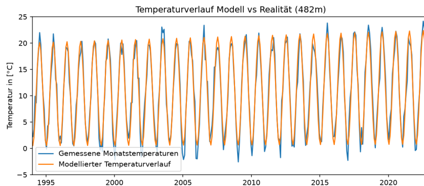
Abbildung 8: Modellerte Temperaturentwicklung vs Daten von 1994 bis 2023
