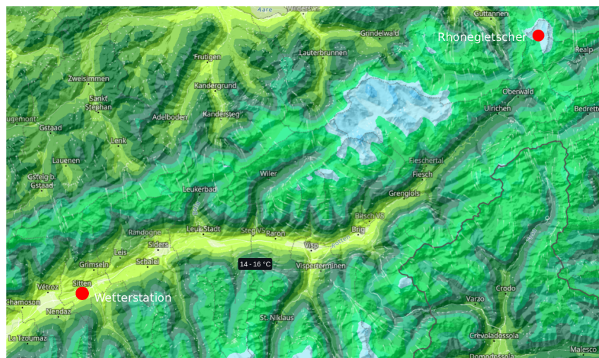
Abbildung 2: Die Entfernung ist jedoch im gleichen Tal („Rezente Temperaturkarte des Rhonetals mit Rhonegletscher und Messstation“, 2026)
