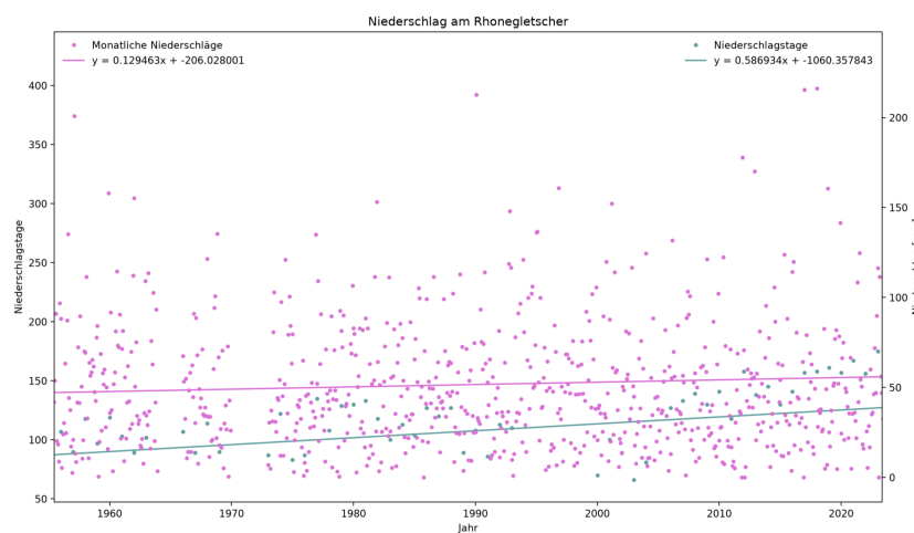
Abbildung 12: Jährliche Regentagsanzahl, monatliche Niederschläge und die Ausgleichsgeraden
