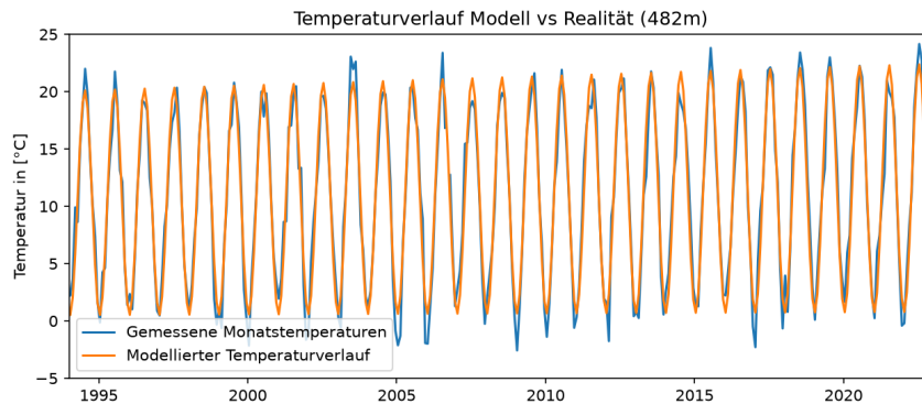
Abbildung 10: Modellierte Temperaturentwicklung vs. Daten von 1994 bis 2023
