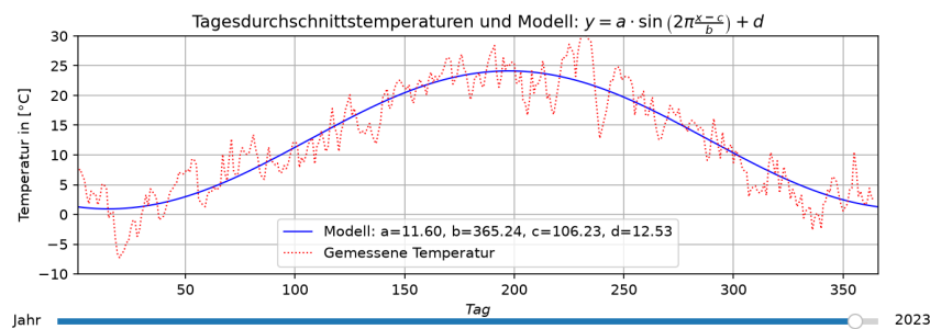
Abbildung 7: Temperatur-Sinuskurve für 2023
