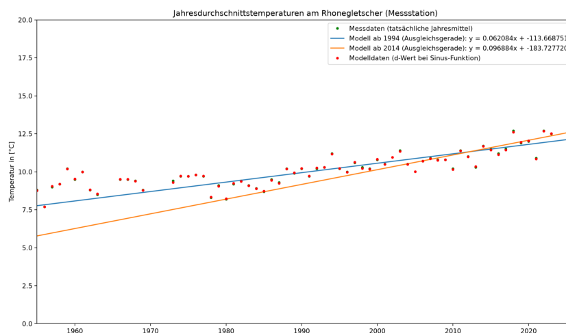
Abbildung 9: Modellierte Temperaturentwicklung mit Daten seit 1994 und 2014
