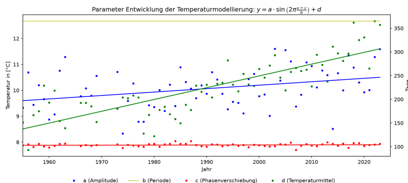
Abbildung 8: Entwicklung der Parameter a , b , c und d
