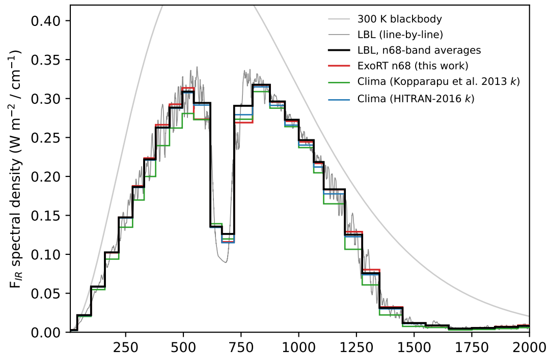
Inner HZ: moist T_s = 300 K (1 bar N_2 + 330 ppm CO_2 + H_2O )
