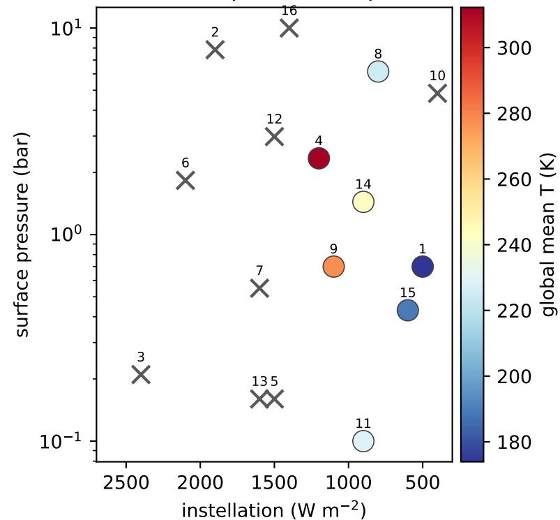
SAMOSA parameter space
