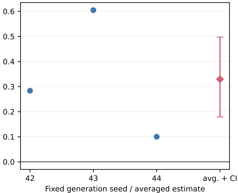
FG-PSNR (dB)
