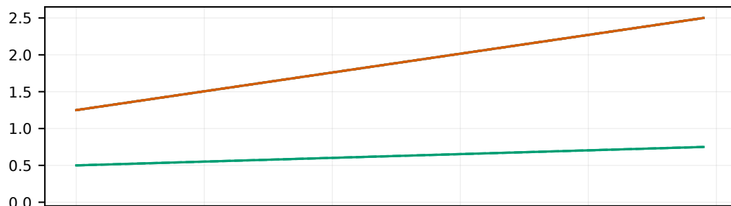
generic linear
