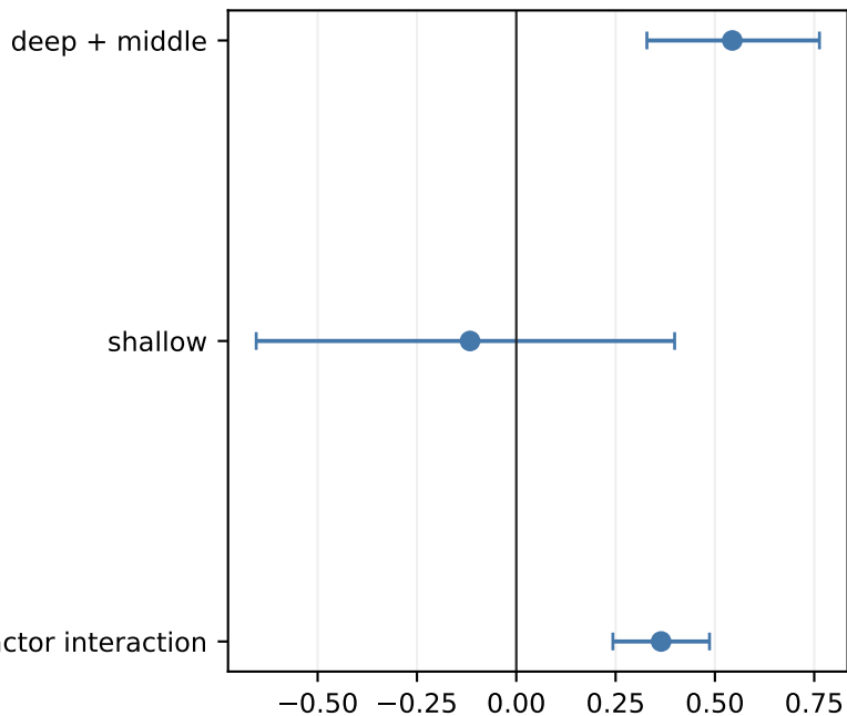
FG-PSNR (dB)
