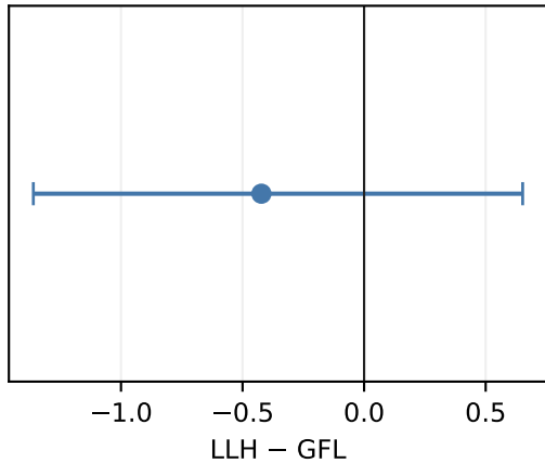
FG-PSNR (dB)
