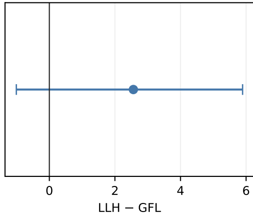
CIEDE2000
