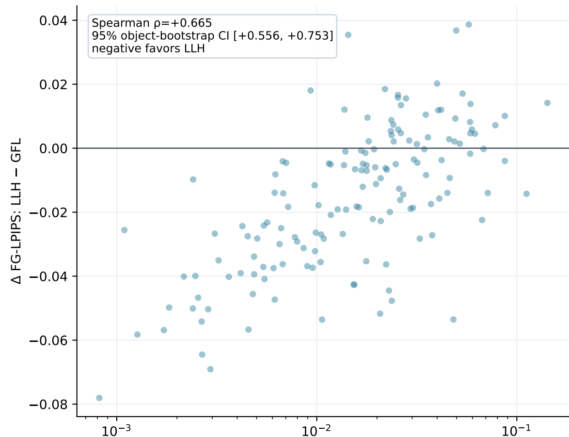
\Delta FG-LPIPS: LLH – GFL
