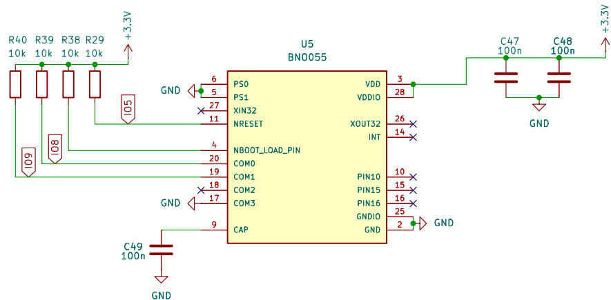
BN0055 IMU
