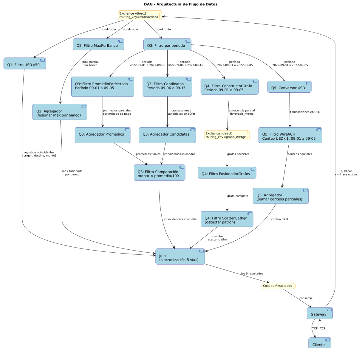
Figura 1: Diagrama D.A.G.
