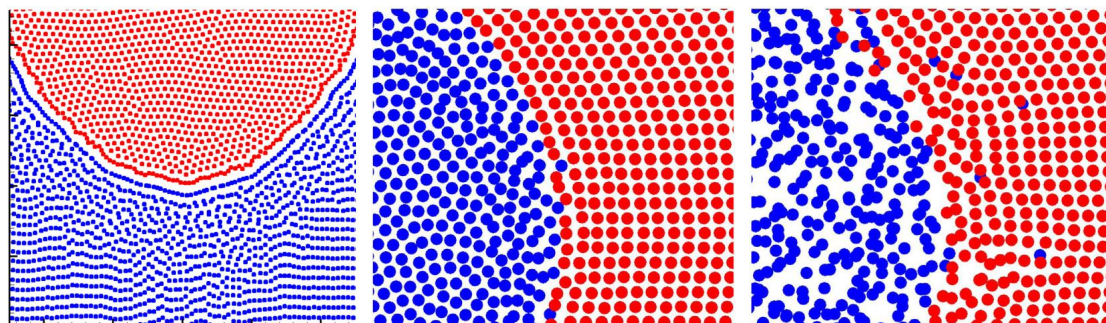
图 2. 不可压-可压 SPH 两相界面。左：保持真实物性比以及清晰界面 [24] ；中右：高物性比及表面张力处理不当引起界面混粒 [30]
