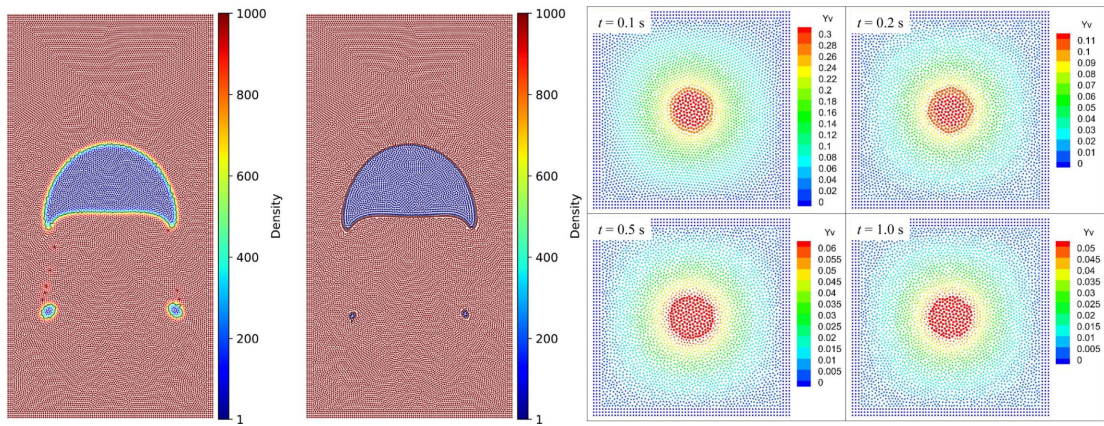
图 3. SPH 相变建模界面特征。左：扩散界面与清晰界面 [31] ；右：扩散界面 [47]
