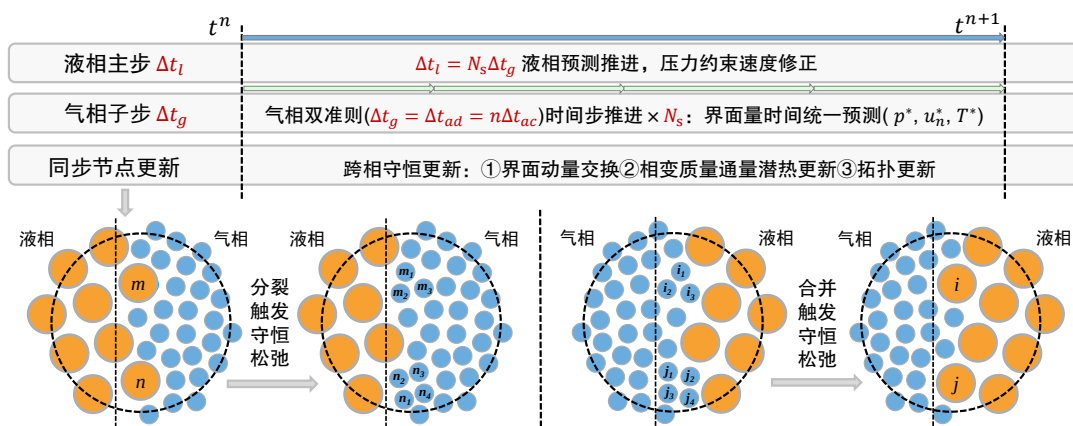
图 10. 同步节点下跨相同层更新与拓扑更新嵌入示意
