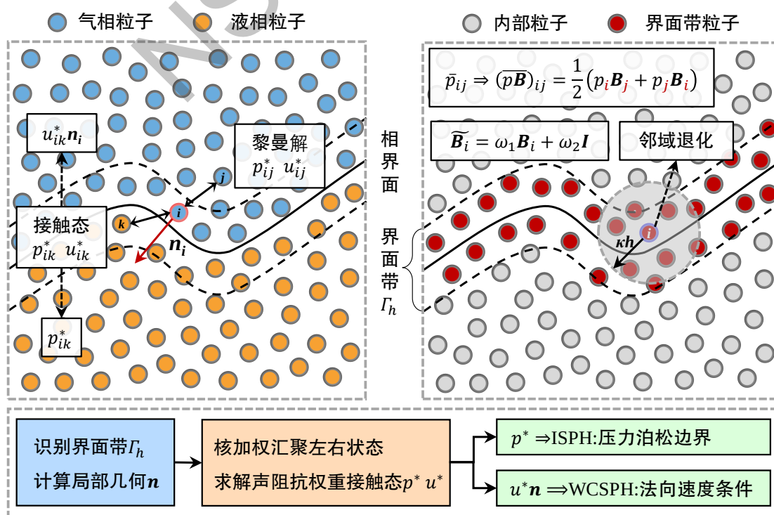
图 8. 界面带共享接触态的两相同层耦合方法
