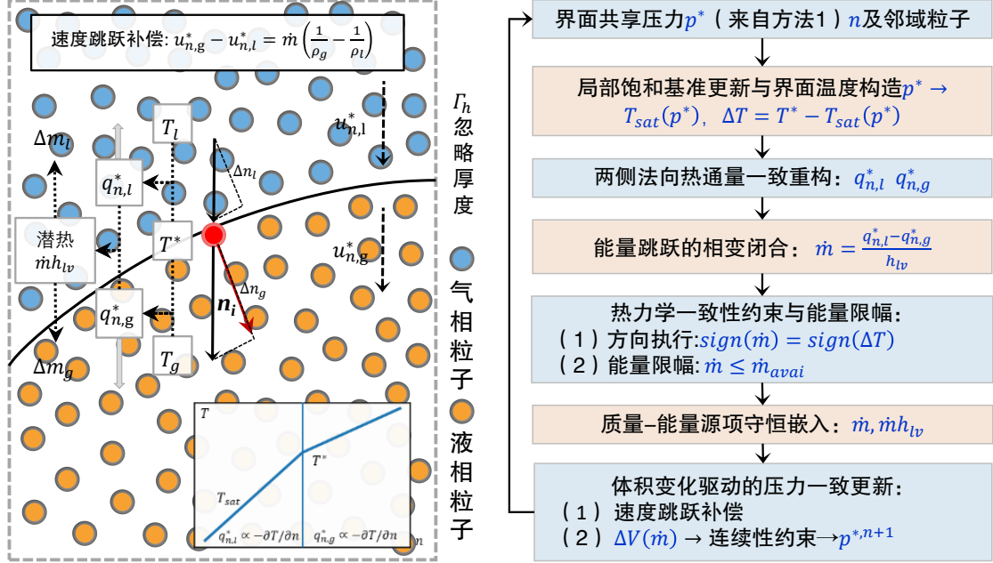
图 9. 热通量驱动的两相闭合并潜热守恒更新流程
