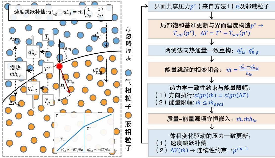
图 8. 热通量驱动的质量通量离散与潜热守恒更新流程
