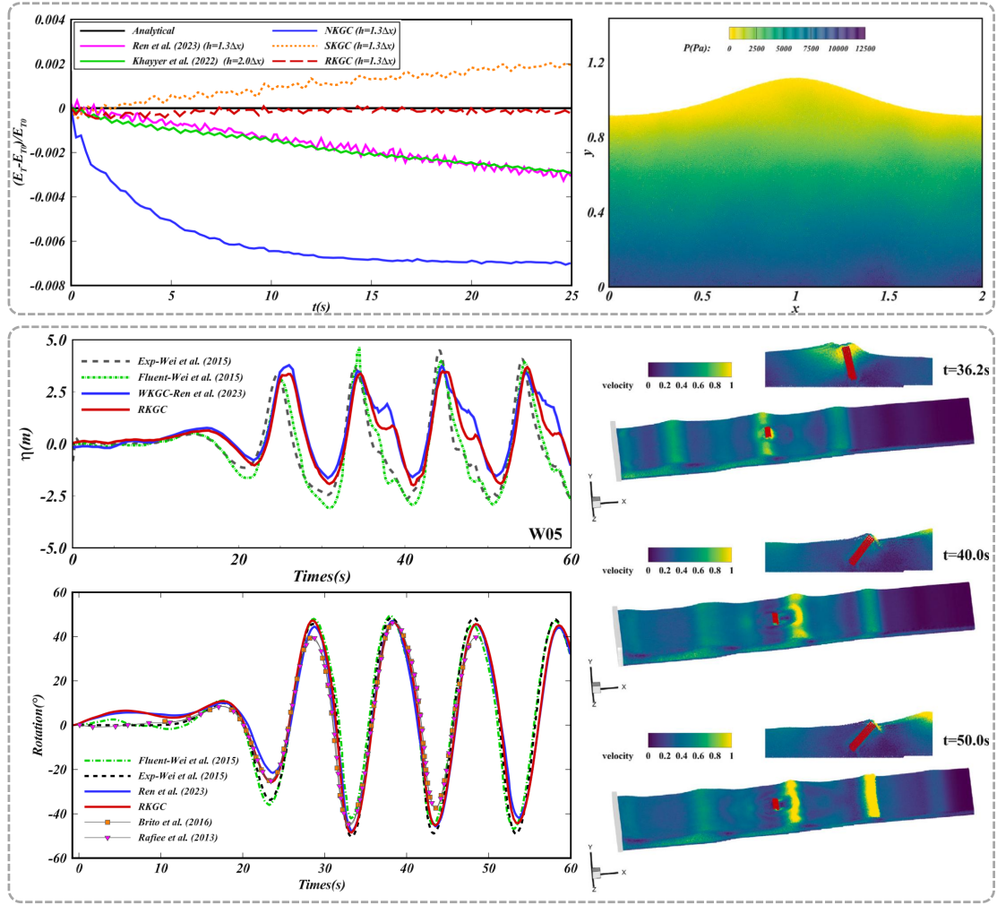
图 10. 守恒高阶一致性离散工作基础。上：驻波算例的能量耗散对比与压力云图；下：波浪能量转换装置算例的定量对比与速度云图
