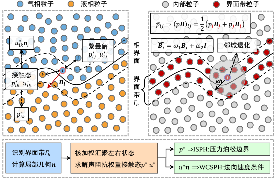
图 7. 界面带共享接触态的两相同层耦合方法
