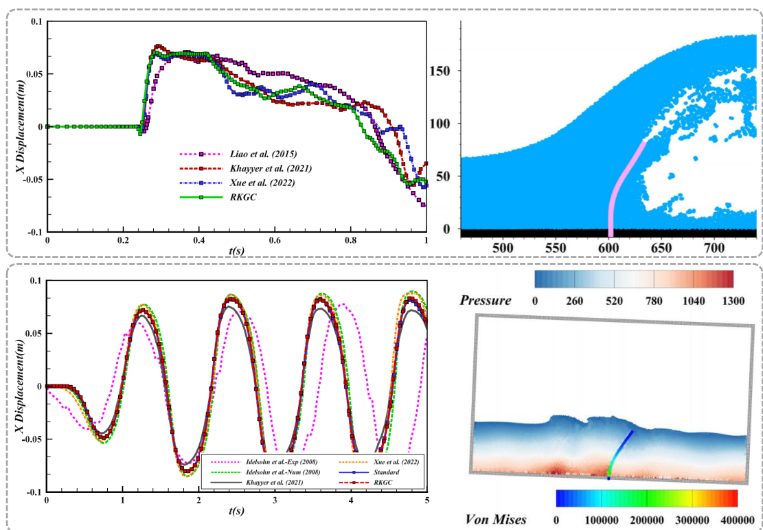
图 12. 修正黎曼多分辨率流固耦合工作基础。上：溃坝水流冲击弹性板的对比与结果验证；下：带弹性挡板滚动水箱晃动算例的对比与结果验证
