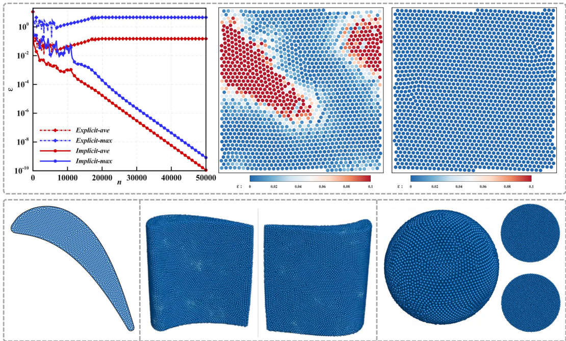
图 14. 粒子松弛工作基础。上：隐式粒子松弛收敛特性；下：复杂几何粒子生成
