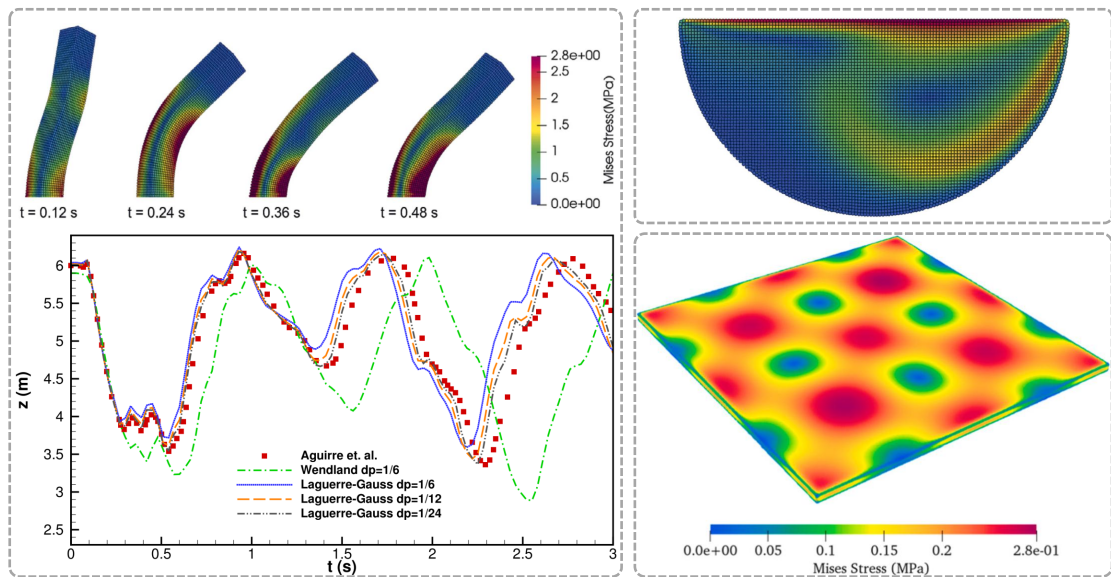
图 11. 高阶核函数检验与应用工作基础。左：三维弯曲柱应力云图及收敛对比；右上：顶盖驱动半圆腔体速度云图；右下：三维振荡板应力云图
