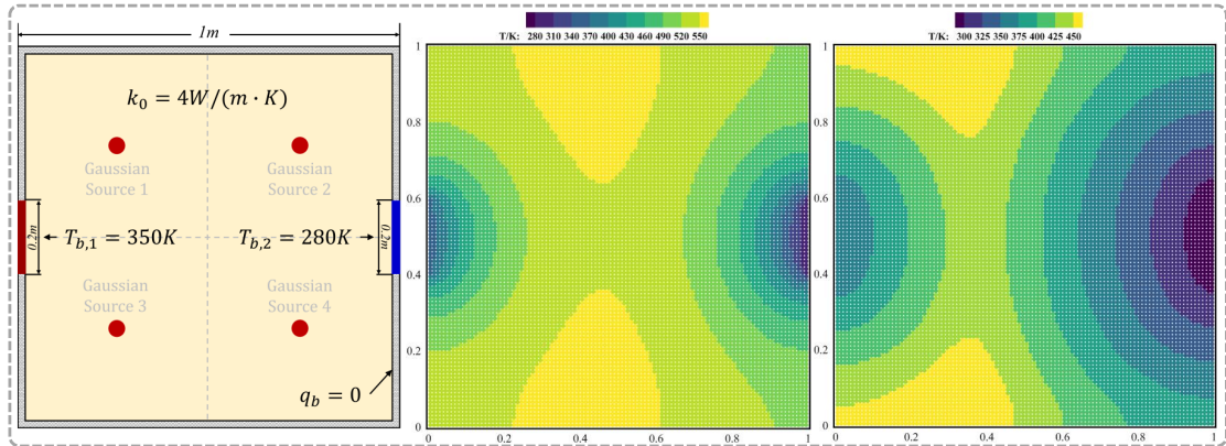
图 13. 传热求解与热边界处理工作基础。左：热边界条件示意；中：均匀热导率下的温度场；右：优化热导率分布下的温度场
