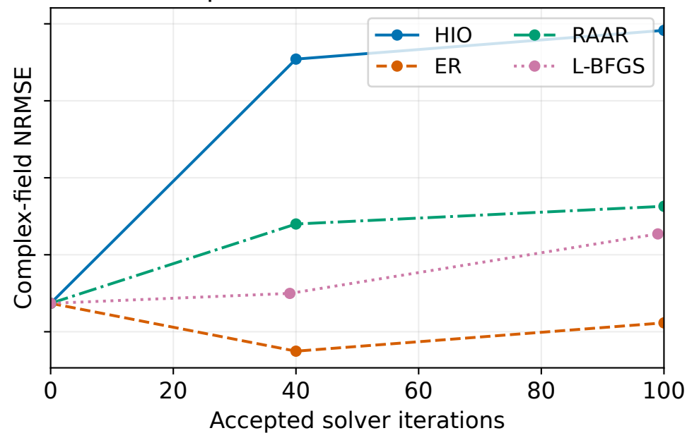
(d) Aperiodic / shot + read noise
