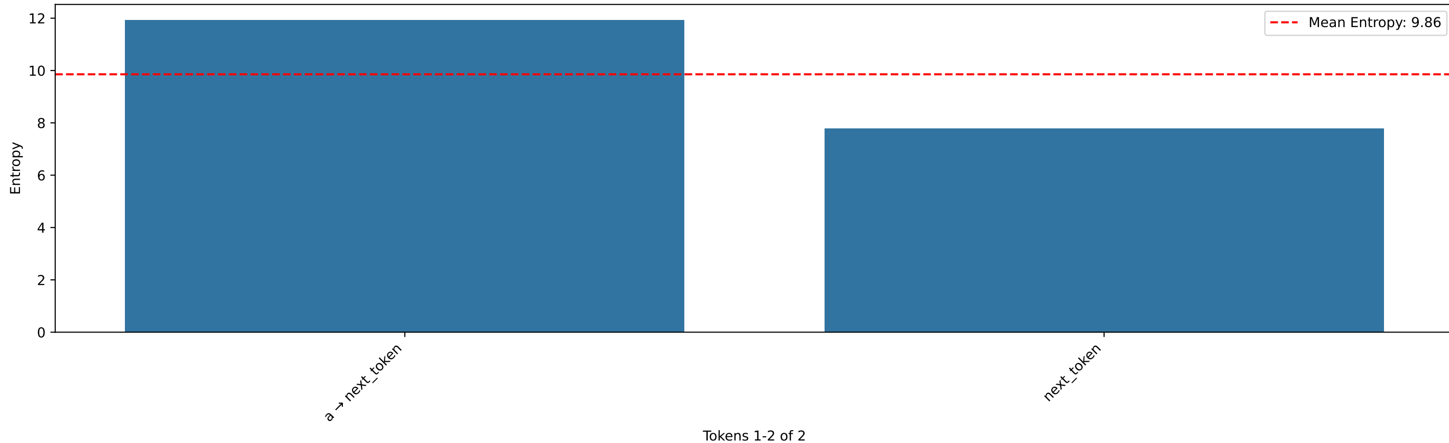
Output Token Entropies (Part 1/1)
