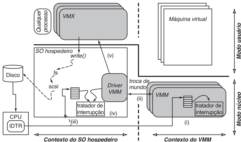
FIGURA 7.10 A VMware Hosted Architecture e seus três componentes: VMX, driver VMM e VMM.
