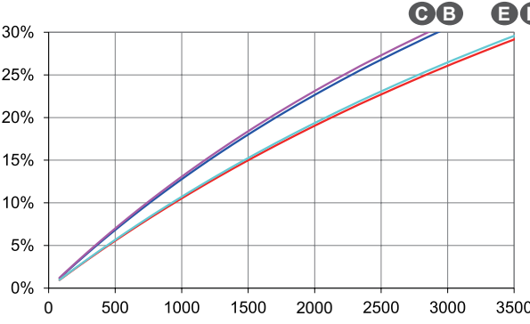
负载突加 (AREP+/PMG) - kVA at 0.8 P.F.
