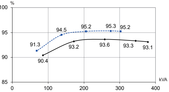
TAL-A46-E - 480V 60Hz
