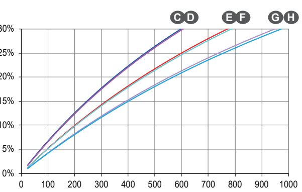
负载突加 (AREP+/PMG)- kVA at 0.8 P.F.
