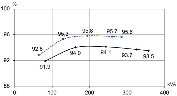
TAL-A46-G - 400V 50Hz
