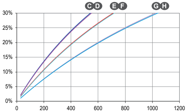
瞬态电压变化曲线 480 V - 60 Hz - 6 & 12线
