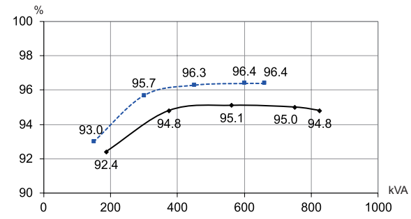
TAL-A473-E - 480V 60 Hz
