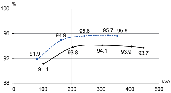
TAL-A46-G - 480V 60Hz
