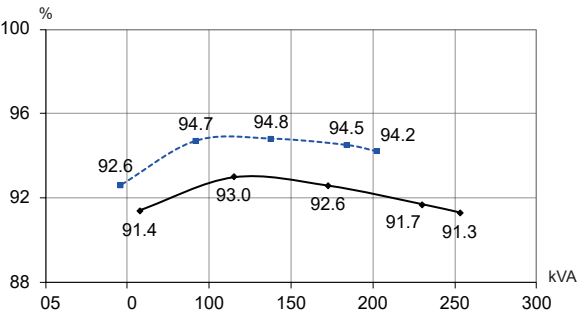
TAL-A46-C - 400V 50Hz
