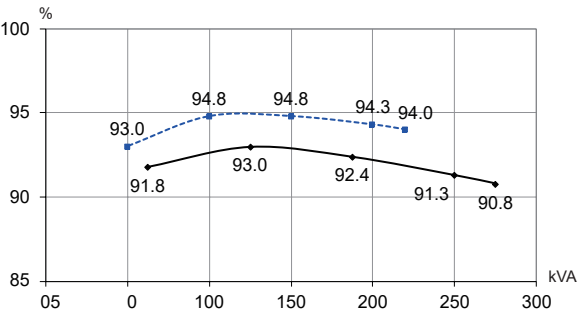
TAL-A46-D - 400V 50Hz
