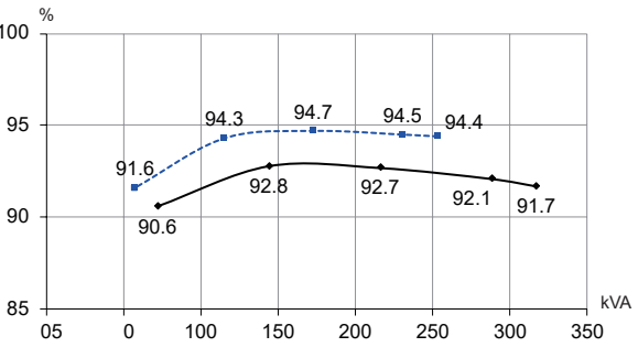
TAL-A46-C - 480V 60Hz
