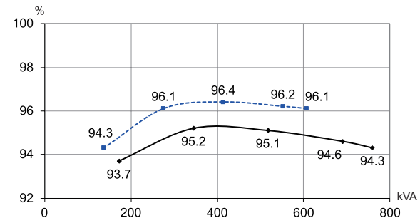
TAL-A473-D - 480V 60 Hz
