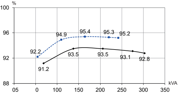
TAL-A46-E - 400V 50Hz
