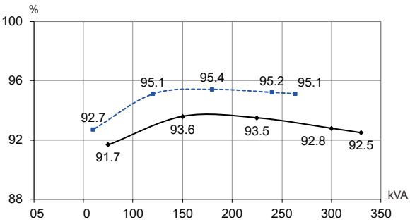
TAL-A46-F - 400V 50Hz
