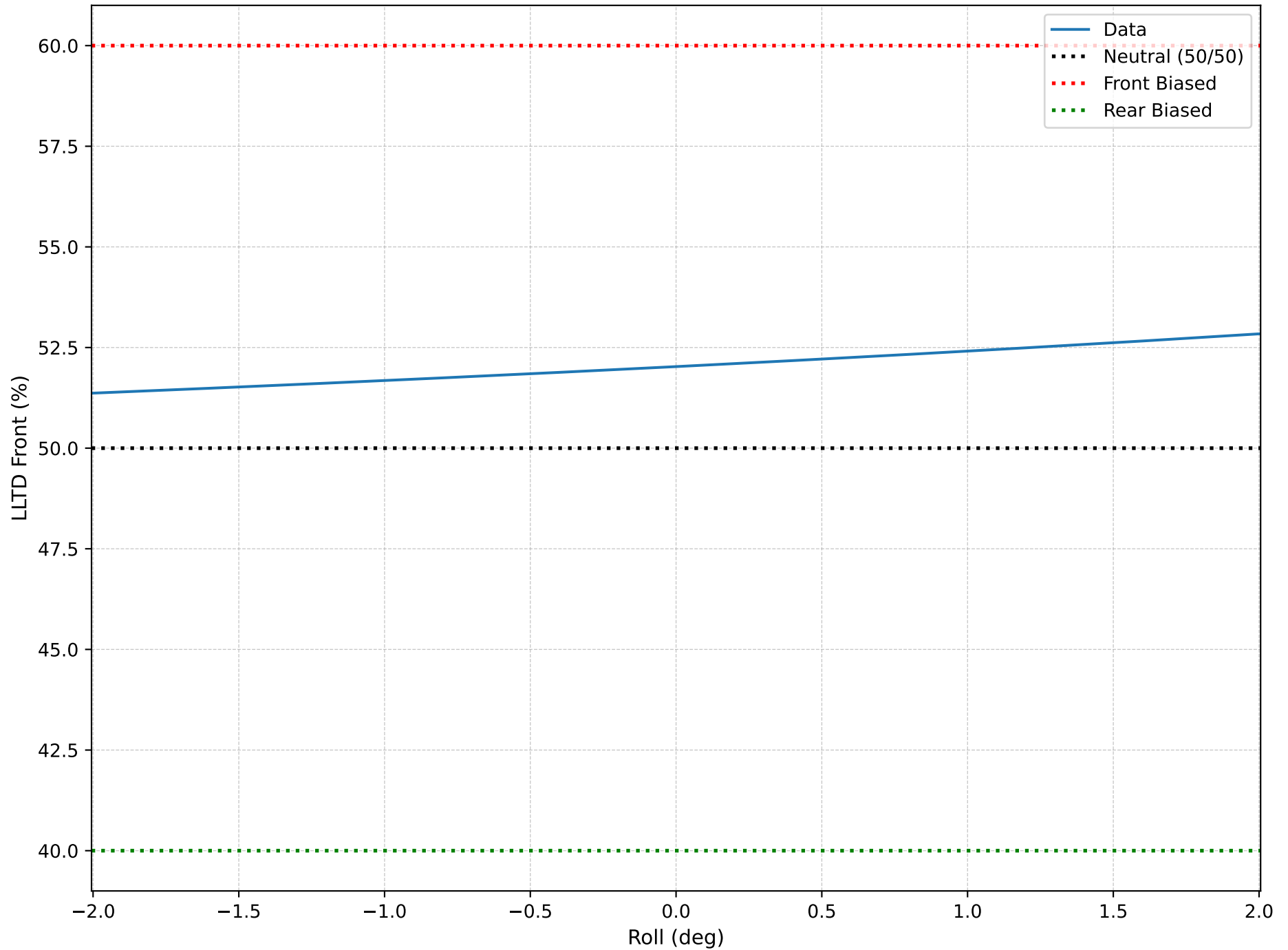
LLTD vs Roll
