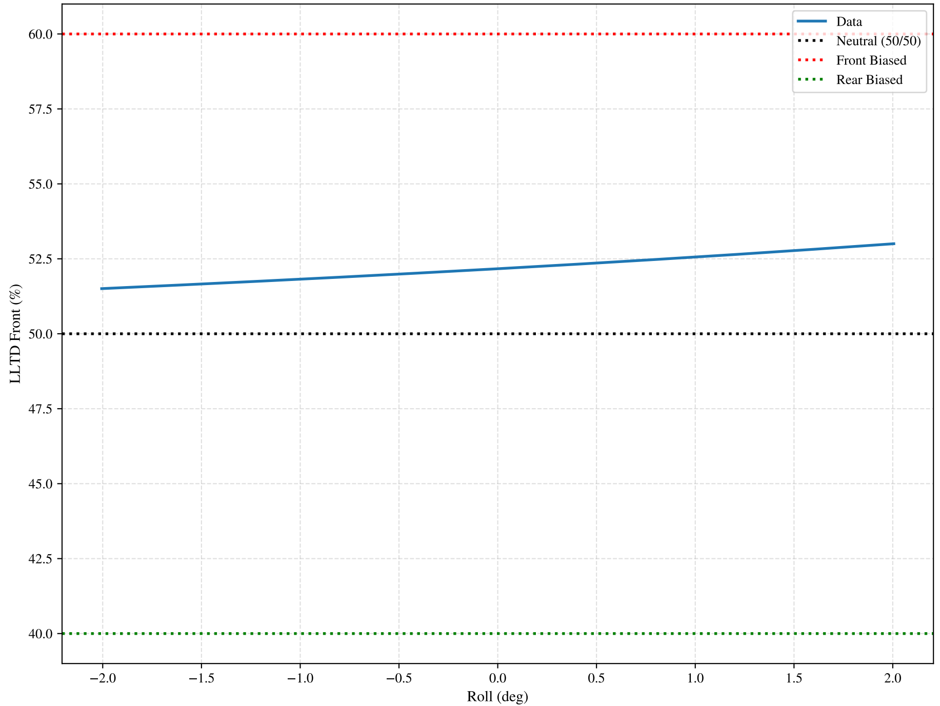
LLTD vs Roll
