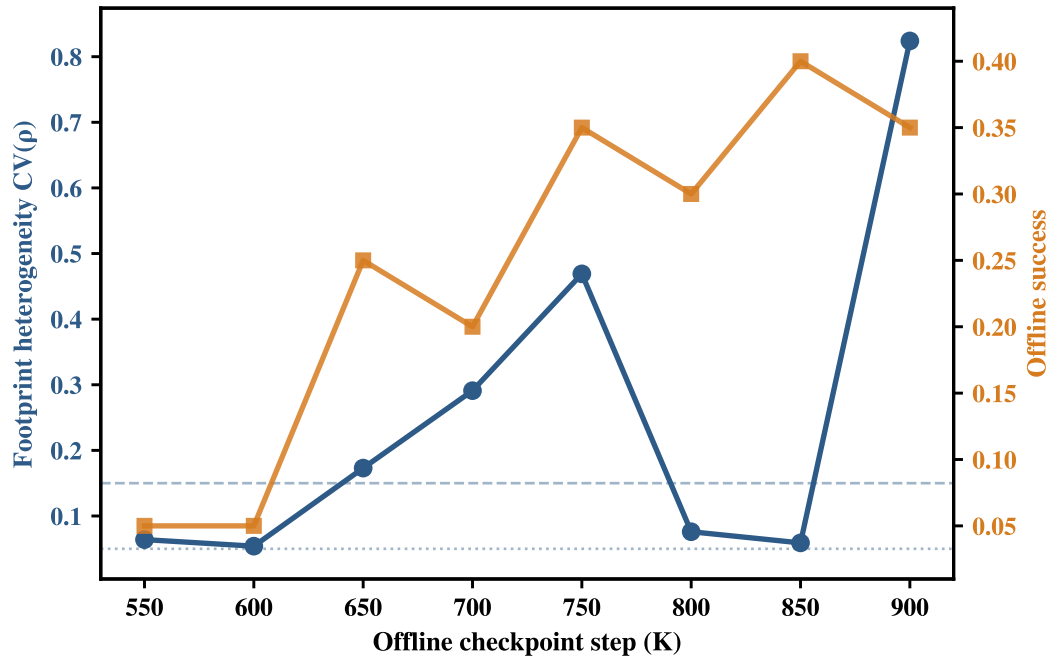
antmaze-large-diverse-v2
