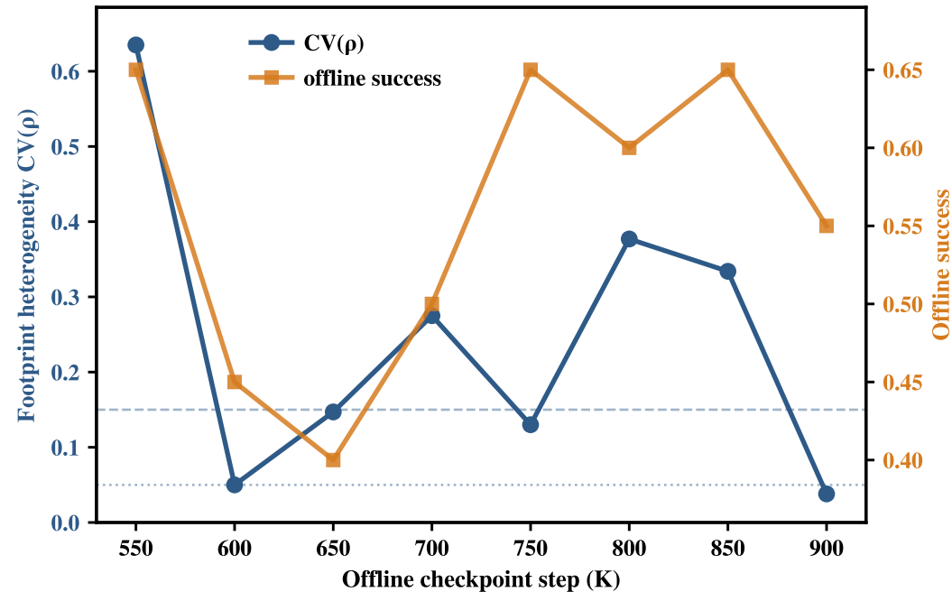
antmaze-medium-diverse-v2
