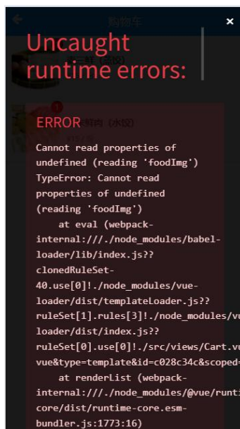
图 8-2 异步请求
