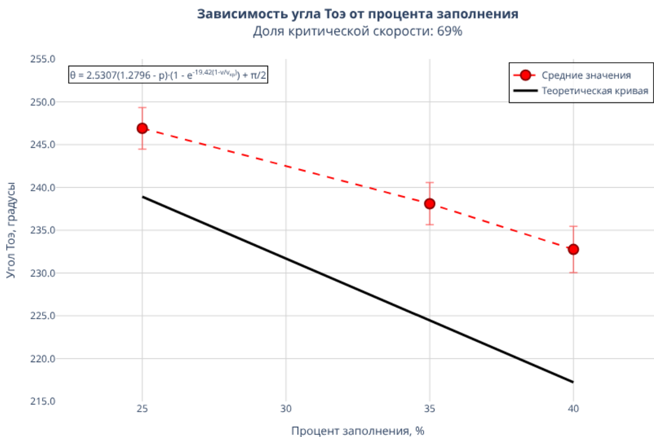
Рис. 3: Зависимость угла Тоэ от заполнения при 69% от критической скорости
