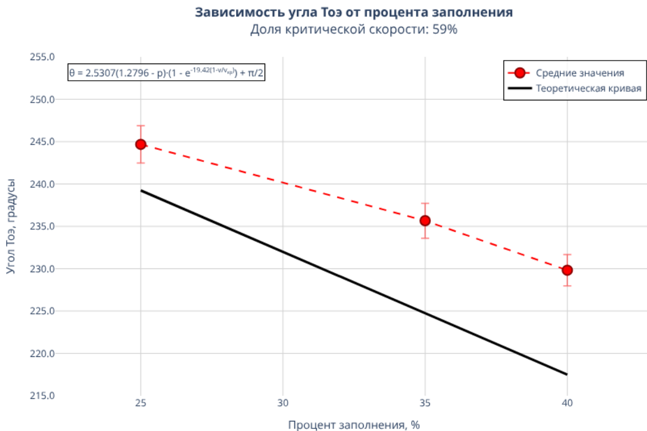
Рис. 2: Зависимость угла Тоэ от заполнения при 59% от критической скорости
