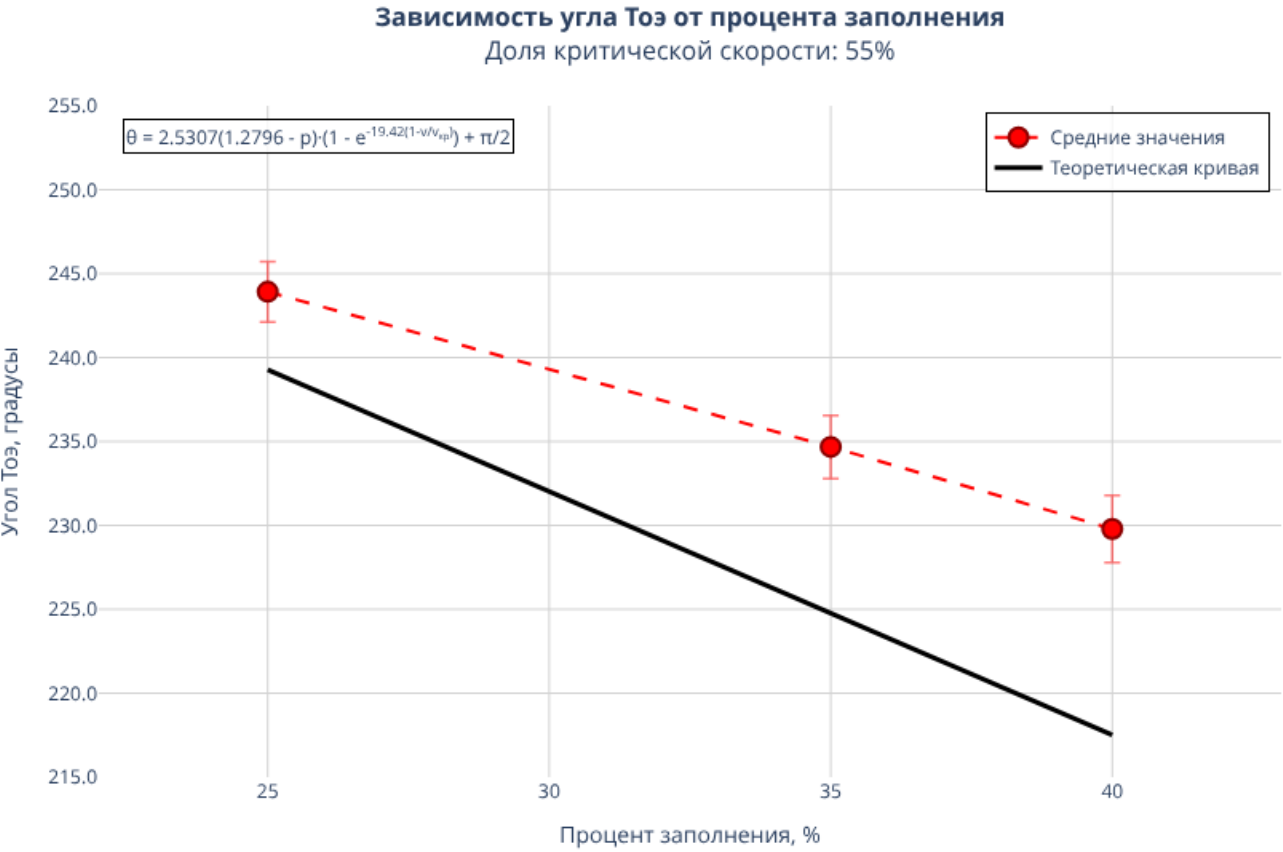
Рис. 1: Зависимость угла Тое от заполнения при 55% от критической скорости
