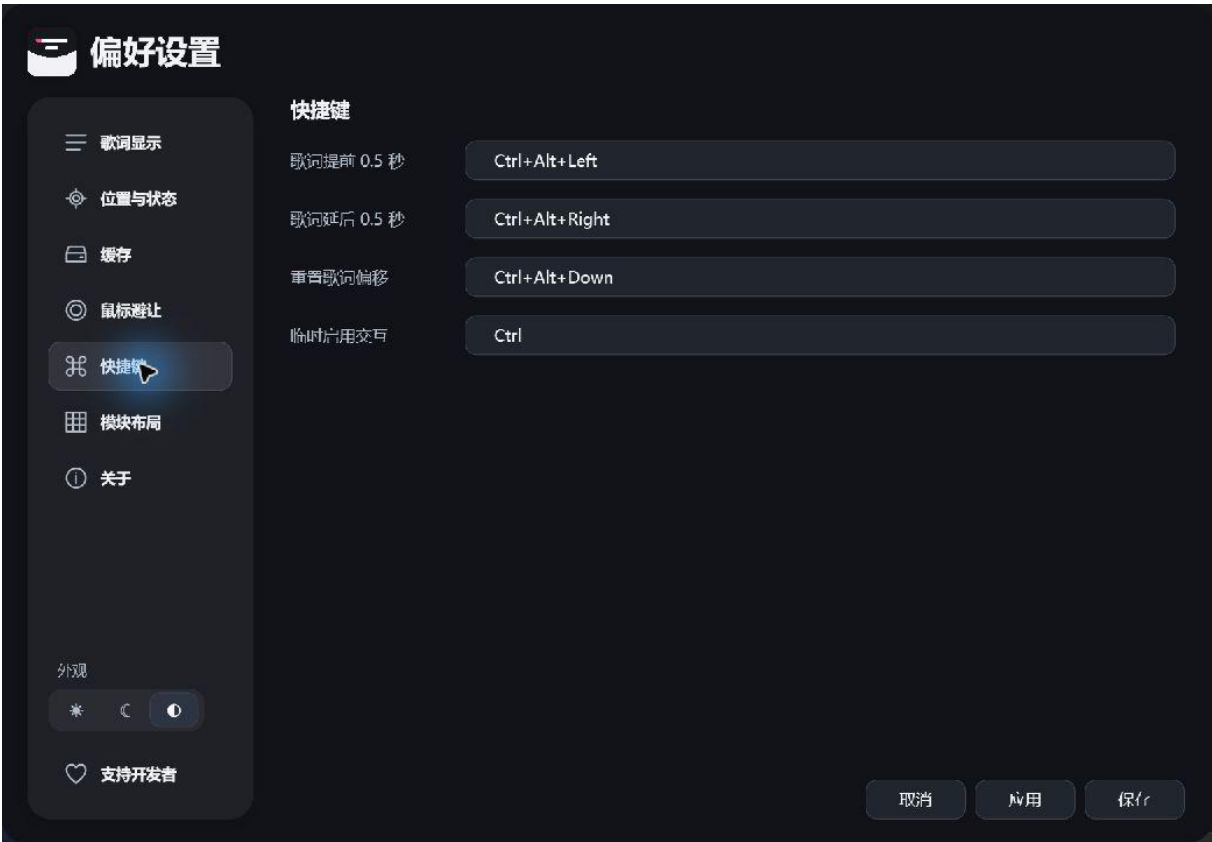
图 6 快捷键设置：提前、延后、重置与临时交互
