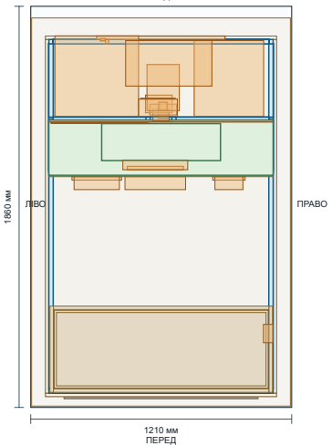
ВИД ЗВЕРХУ
