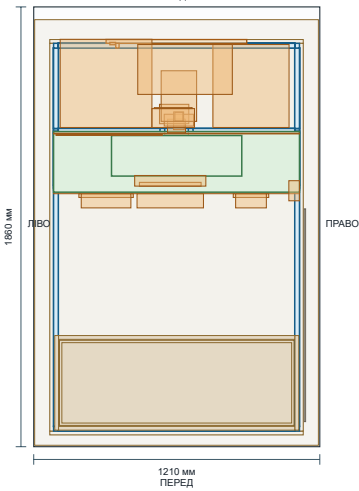
ВИД ЗВЕРХУ
