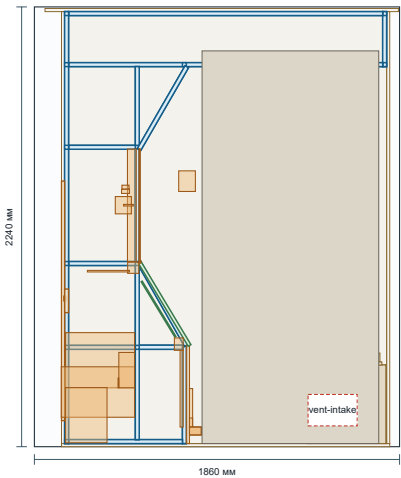
ВИД ЗЛІВА · Y=1072
