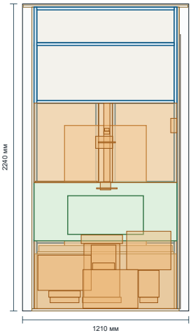
ВИД ЗЛІВА · Y=1072
