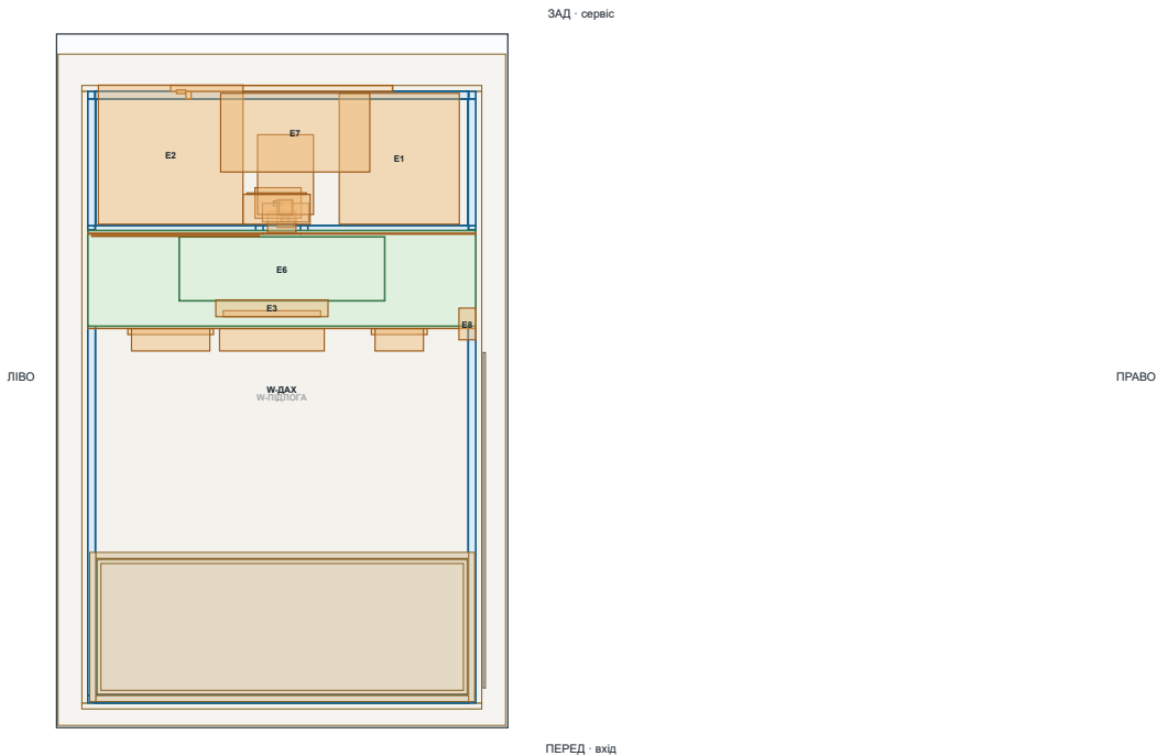
Вид зверху · монтажний план ПЕРЕД унизу (X=0), ЗАД угорі (X=1672), ПРАВО праворуч (Y=0), ЛІВО ліворуч (Y=1072).
