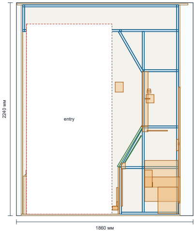
ВИД ЗНИЗУ (план підлоги)
