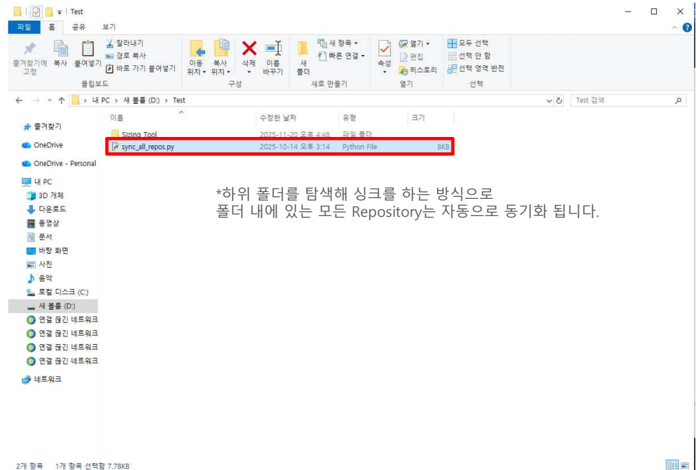
Fig. 5 Python 위치
