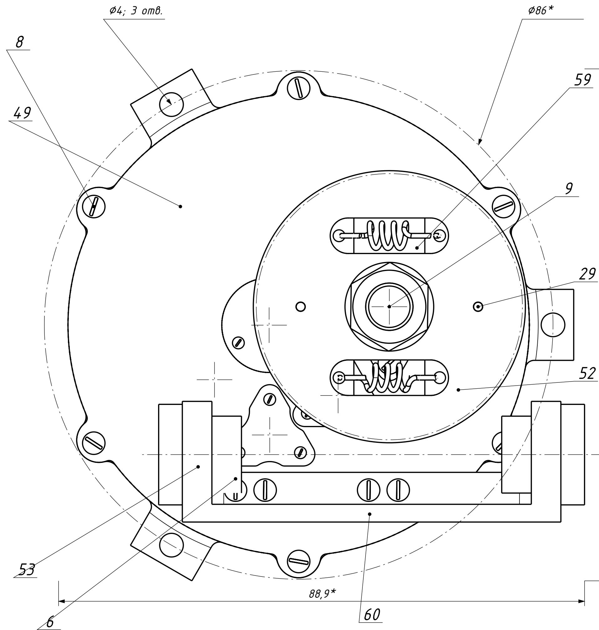
Г-Г (2,5:1)
