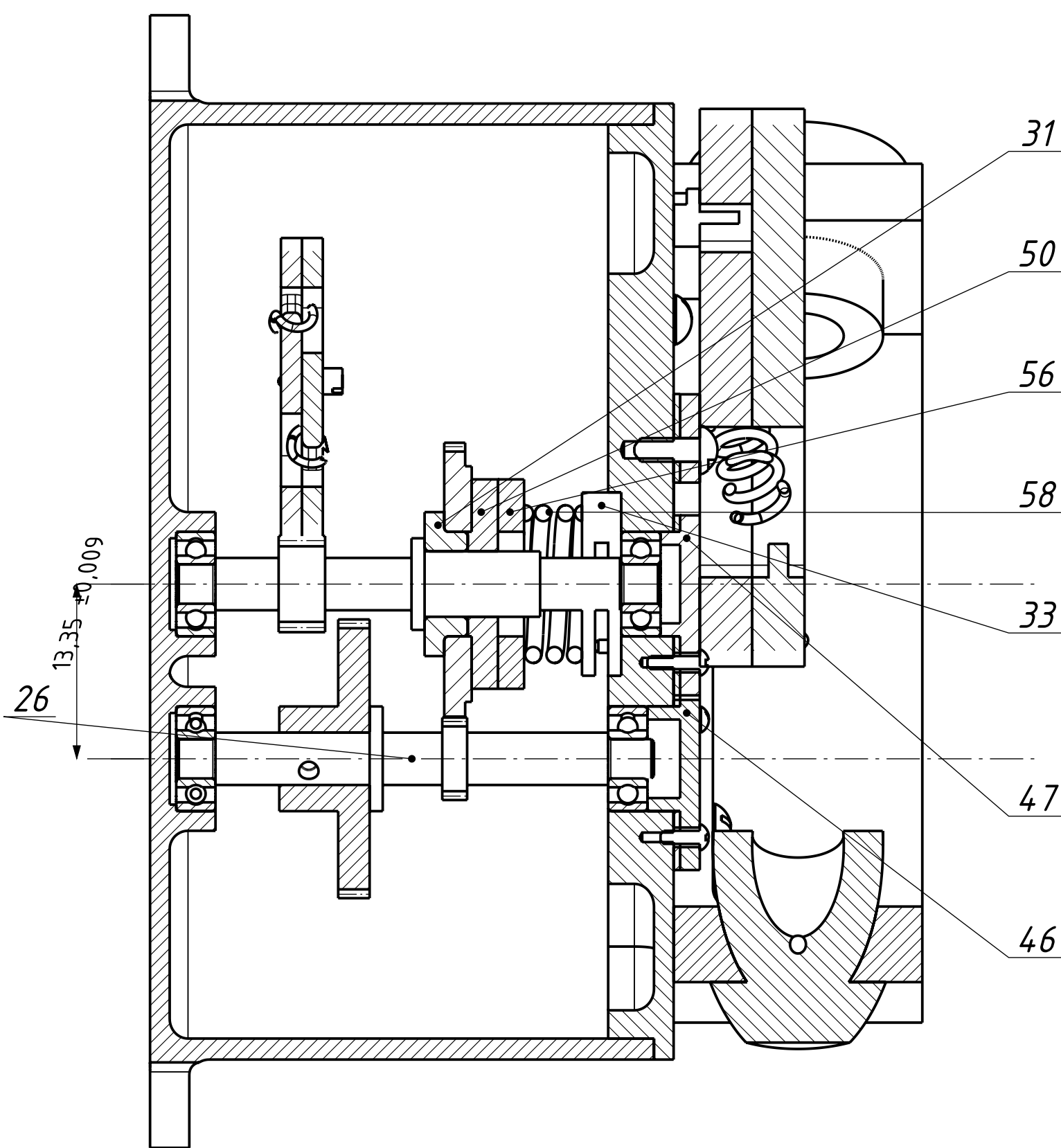
Г-Г (2,5:1)
