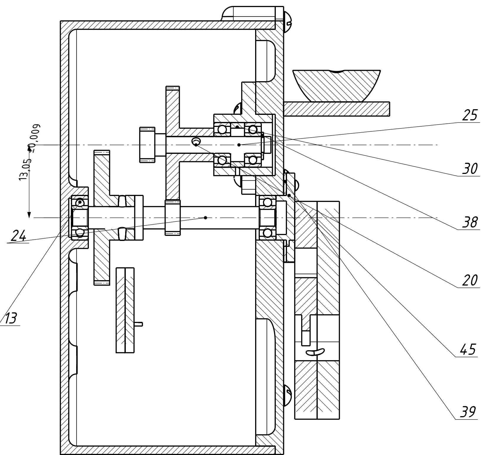
Б-Б (2,5:1)
