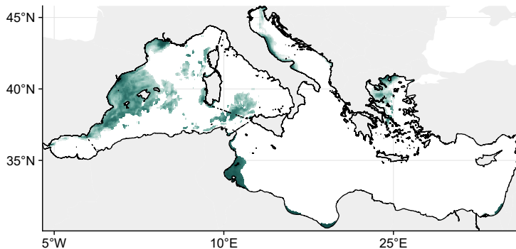
(d) Low Climatic Displacement: Pareto depth
