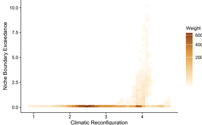
(d) Metric distributions
