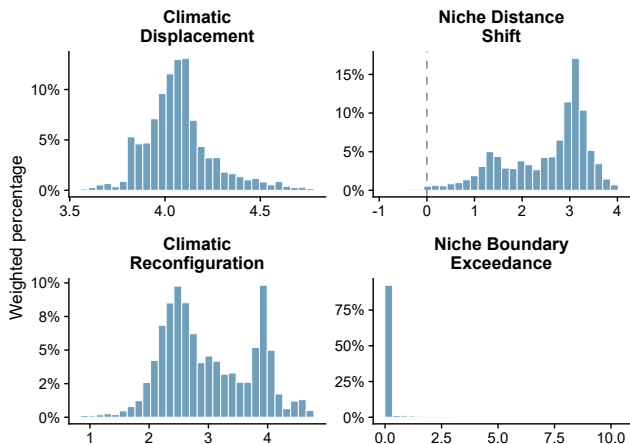
(d) Metric distributions
