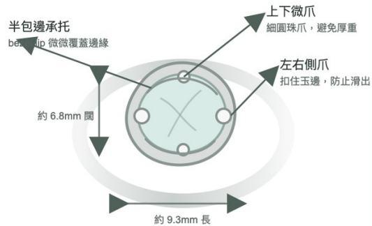
正面 Front View
