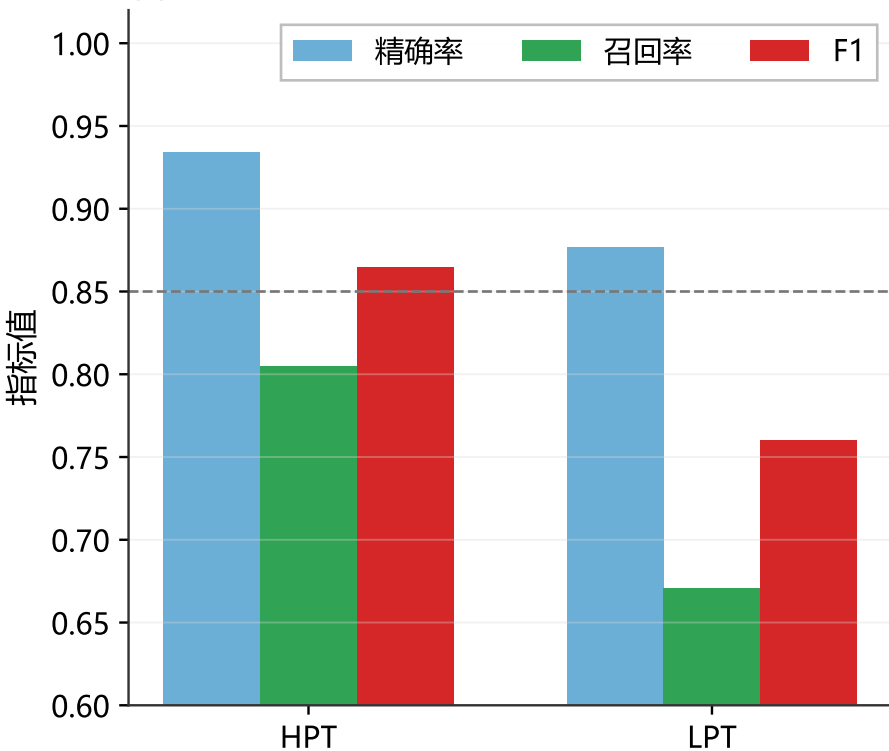
(a) 涡轮内部细分性能
