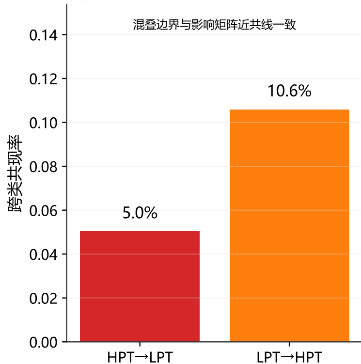
(b) 涡轮内相互混叠
