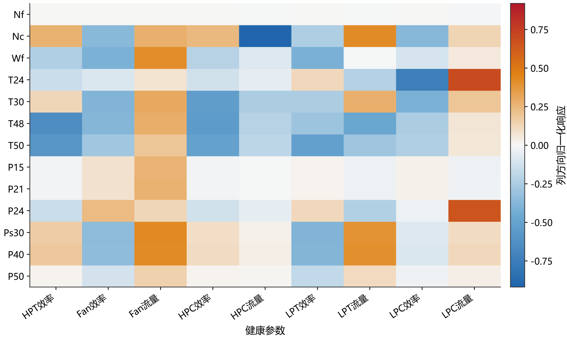
量程归一化影响矩阵的部件故障指纹
