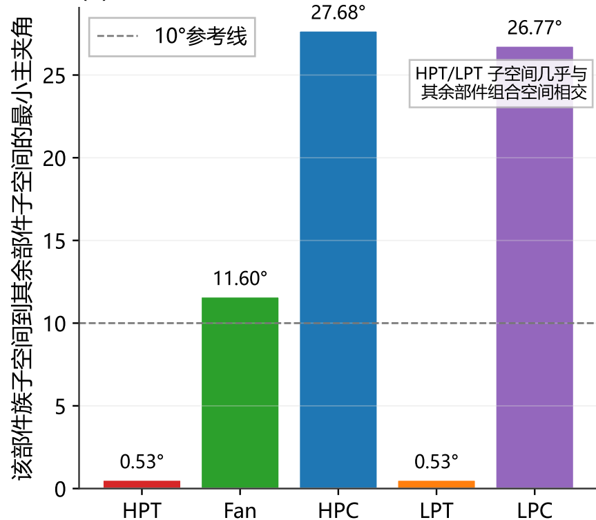
(b) 部件族子空间可辨识性
