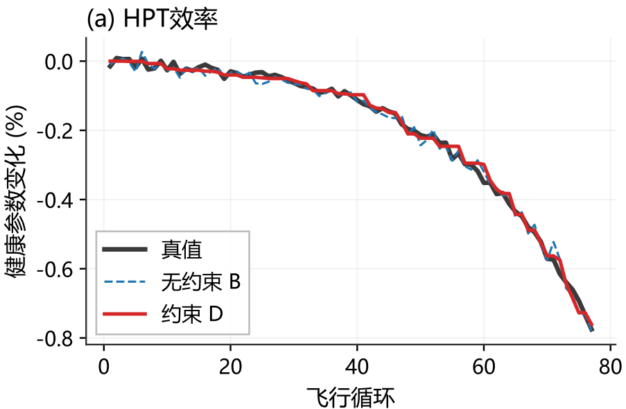
代表发动机连续退化轨迹：相关系数 0.996，RMSE 0.056%
