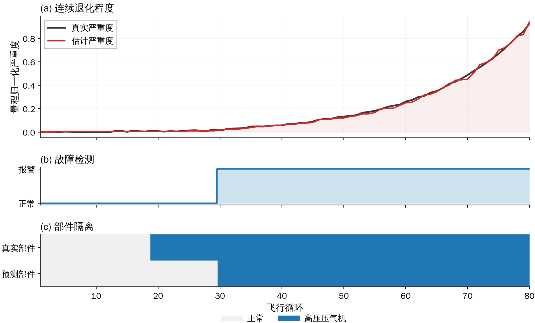
代表发动机从退化出现到部件判定的诊断时间线
